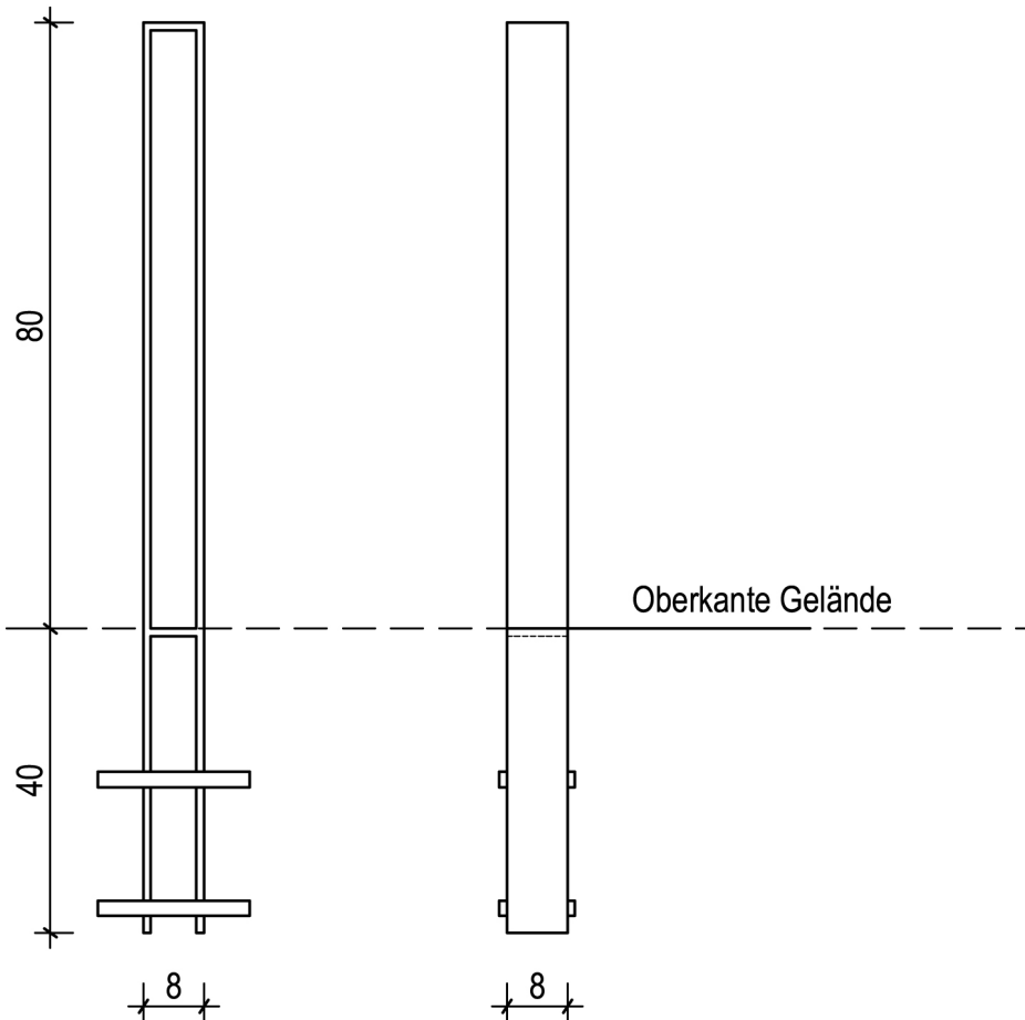
Vorderansicht
